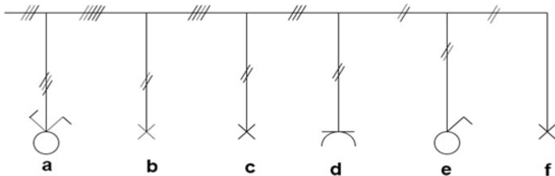
Gambar 3. Single-line diagram praktek instalasi listrik a.Saklar Seri, b.lampu 1 c.lampu 2, d.Stop Kontak, e. Saklar Tunggal dan f. Lampu 3.
